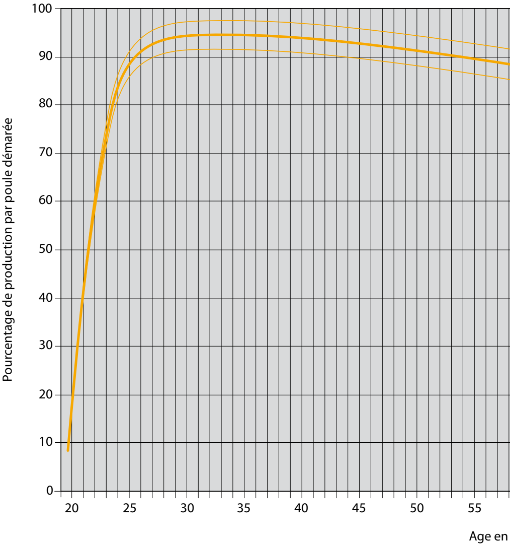
Courbe de production d'œufs des poules pondeuses LOHMANN TRADITION
