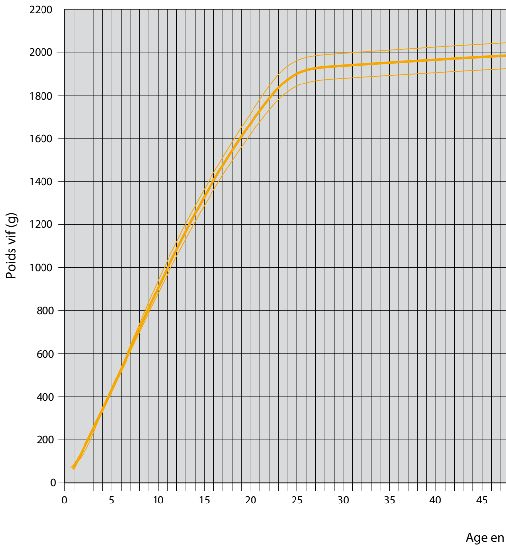
Courbe de croissance de la LOHMANN TRADITION
