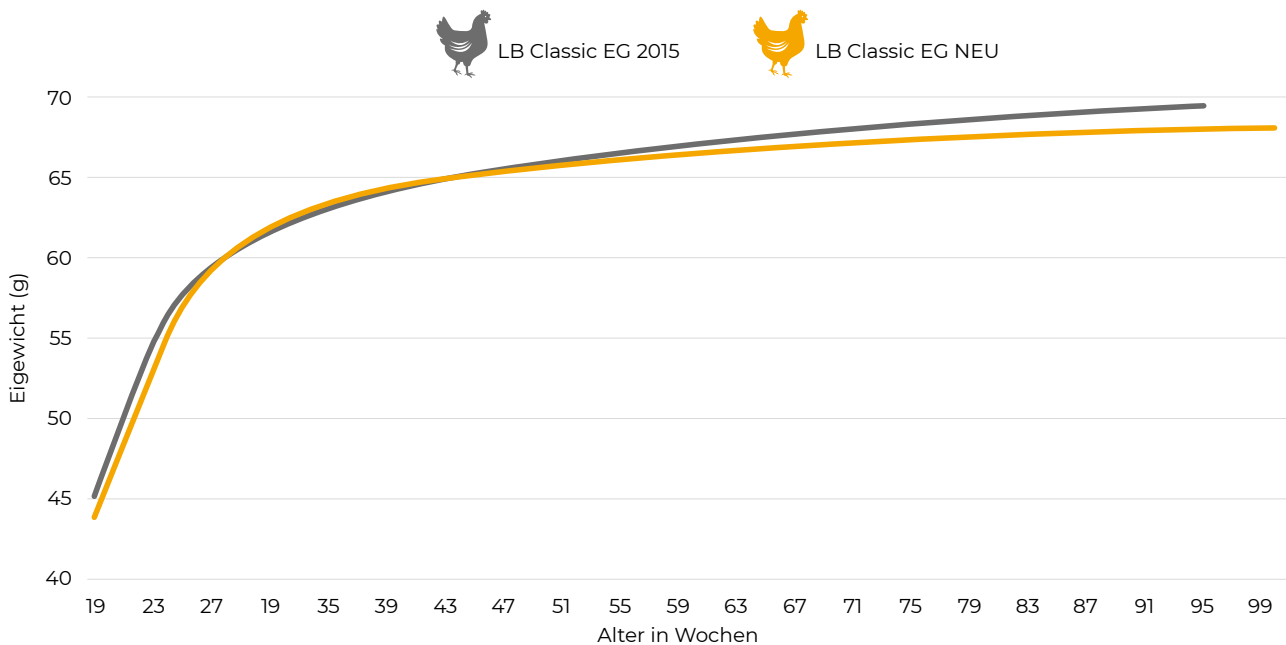
▼ Abbildung 1. Vergleich von alter und neuer Eigewichtskurve (LOHMANN BROWN CLASSIC, Käfigproduktion)
